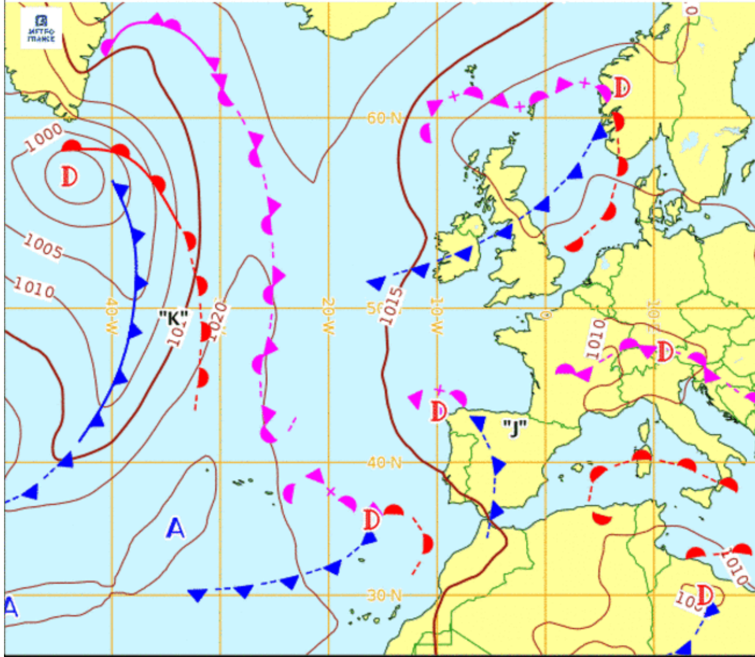
Analyse Fronts et isobares du 26/04/2020 - 12 UTC (reseau: 26/04/2020 - 12 UTC)
